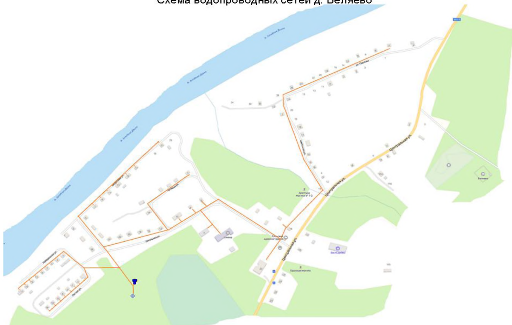
Схема водопроводных сетей д. Беляево
