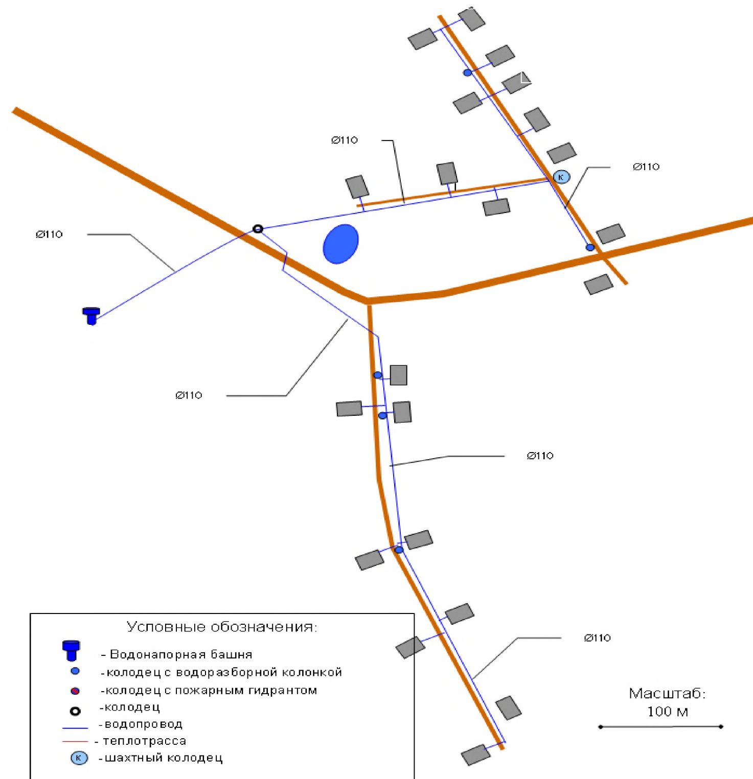
Схема водопроводных сетей д. Патики Чепельские
