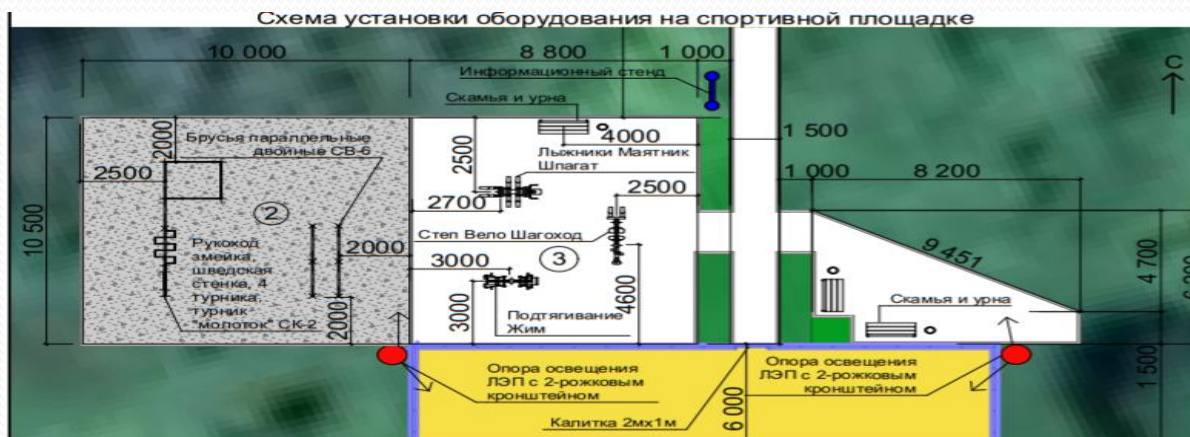
Устанавливаемое оборудования
